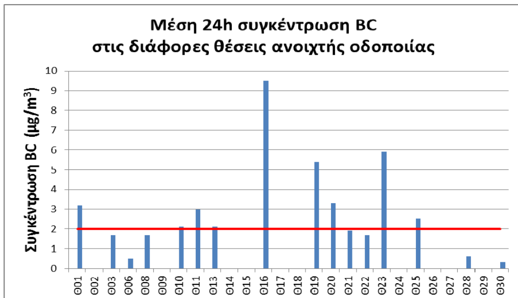
Διάγραμμα 3: Συγκέντρωση BC στις θέσεις ανοιχτής οδοποιίας
